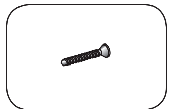
Tornillo conjunto Rotor Silhouette® P.View (CÓD. COSITOR009)
